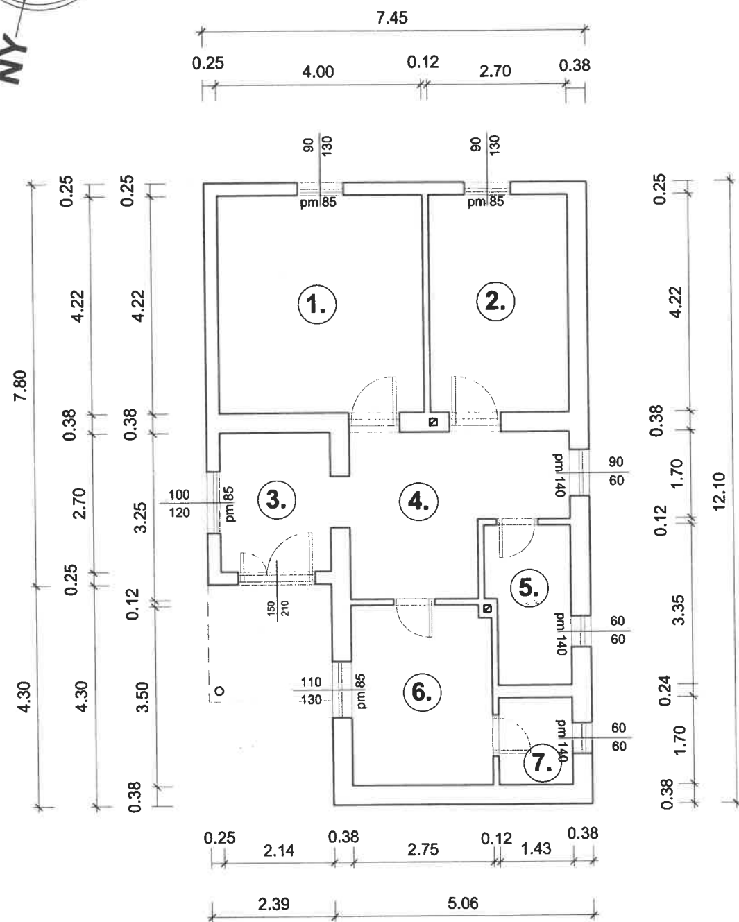
ALAPRAJZ M = 1 : 100
