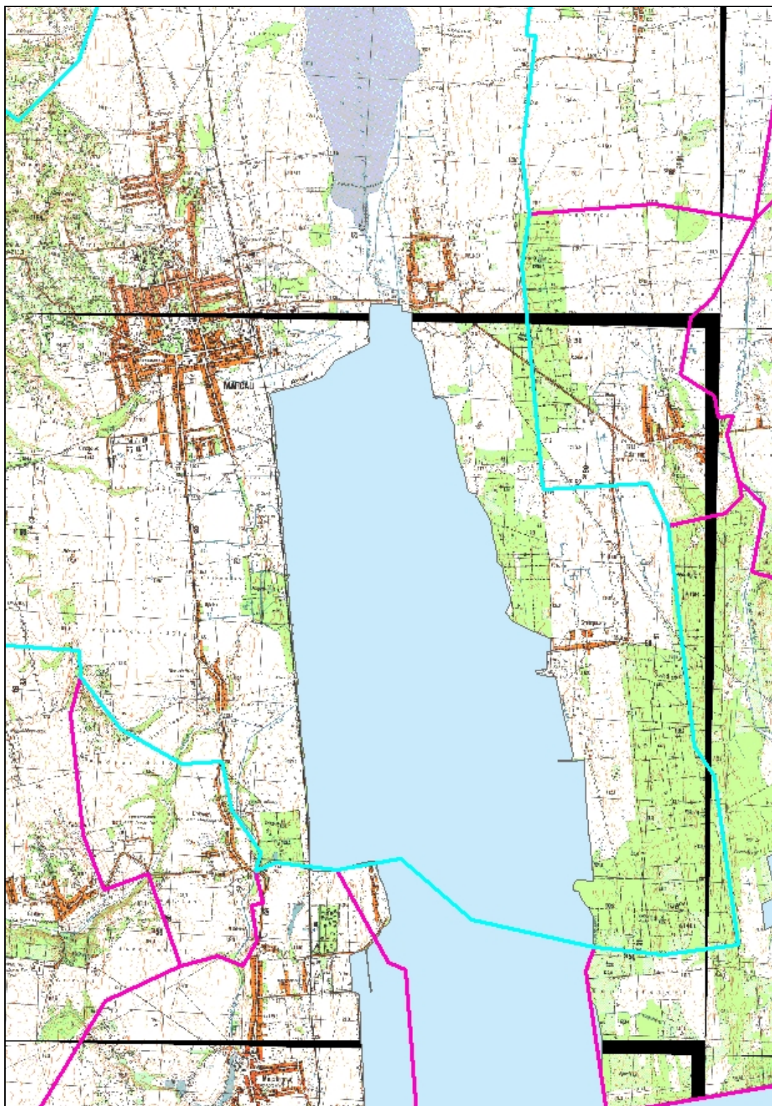
1.13-15. ábra: A Boronka-melléki TK elhelyezkedése Marcali területén (Forrás: DDNPI adatszolgáltatása)
